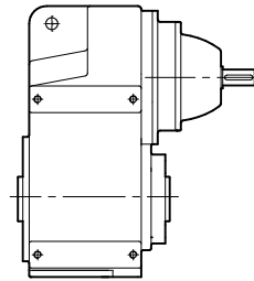
Reduzierstück auf Welle montiert Doppel- / Dreifachreduktion
