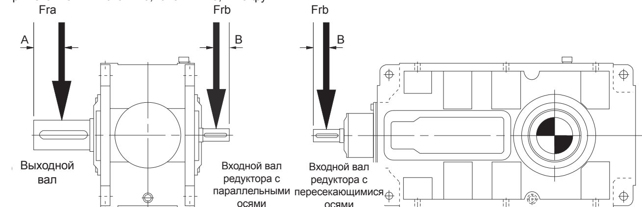
Выходной вал - расстояние 'А' (на середине выступающего конца вала)
