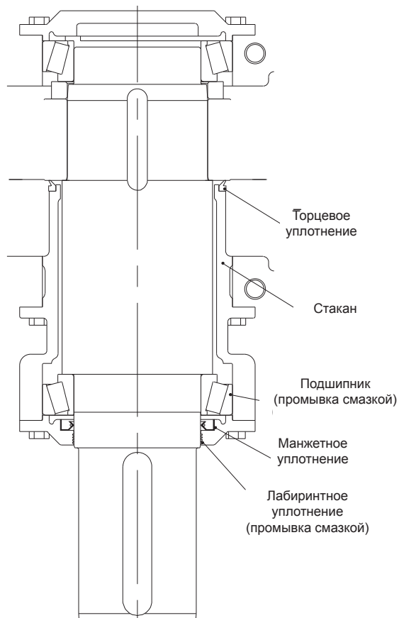
Выходной вал редуктора башни для тяжелого режима работы
