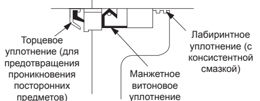
Выходной вал стандартного редуктора
