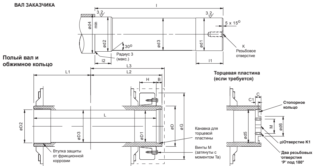
ВАЛ ЗАКАЗЧИКА
