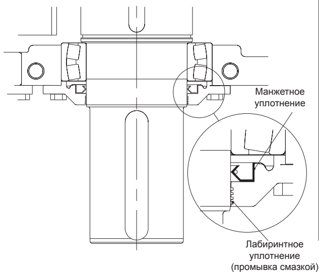
Выходной вал стандартного редуктора
