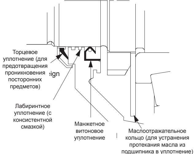
Входной вал редуктора с параллельными осями
