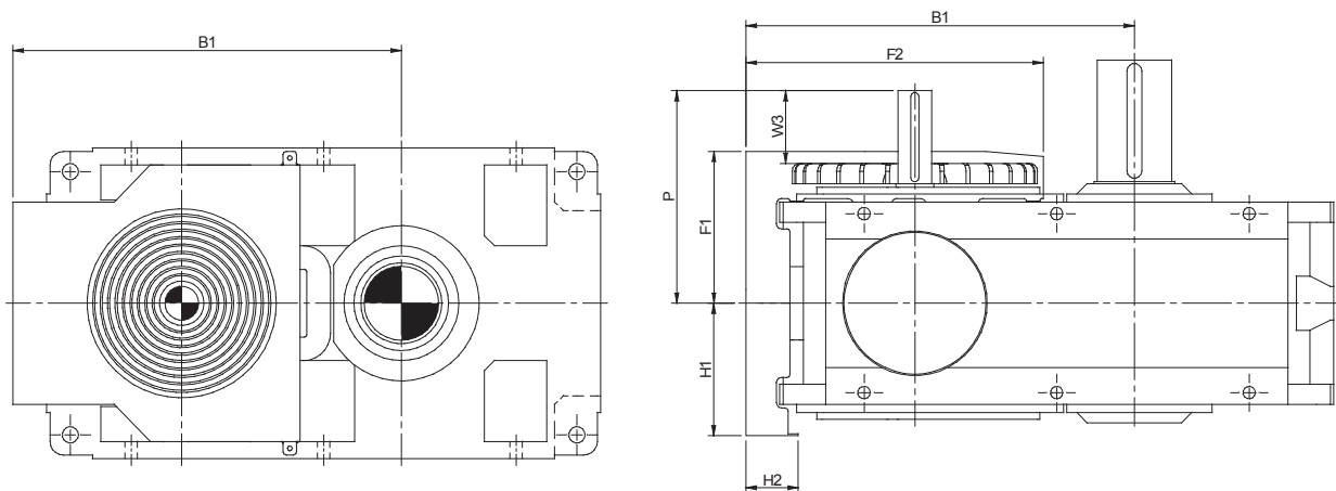
Двухступенчатый редуктор
