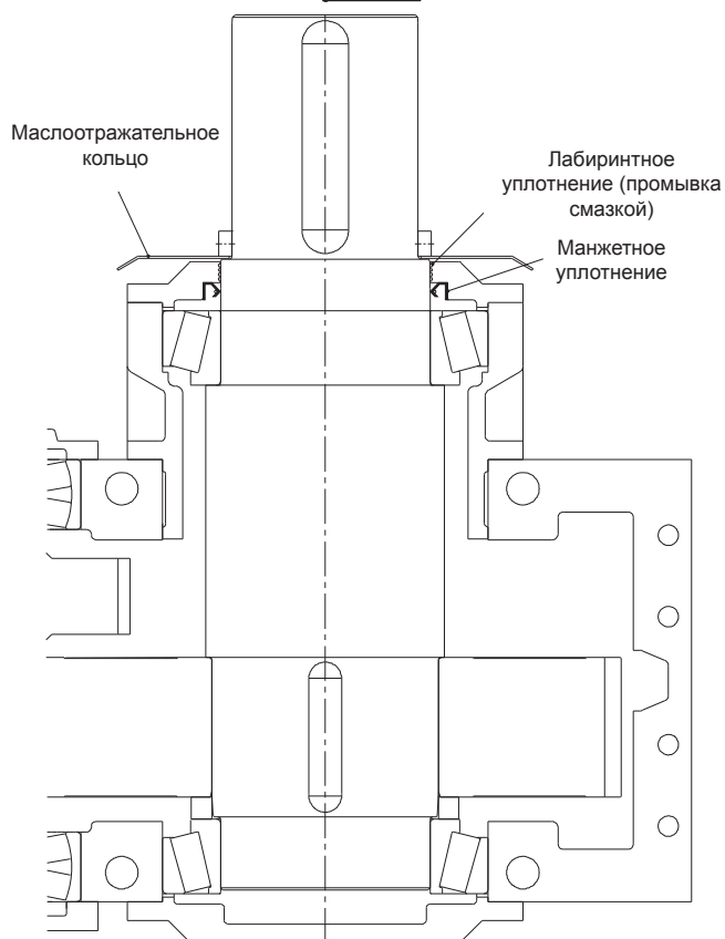
Выходной вал редуктора башни для тяжелого режима работы
