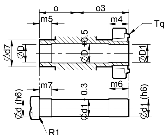
Manchon d'accouplement
