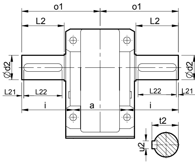
Arbre sortant double
