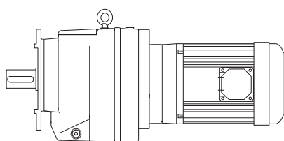
Drei Stufen, Flanschmontage, mit Motor
