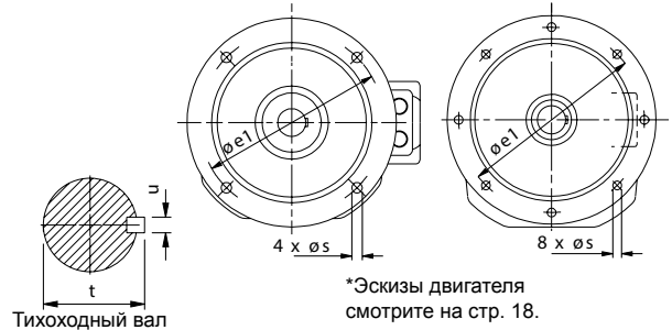
Типоразмеры 1, 2, 3, 4, 5, 6, 7 и 8
