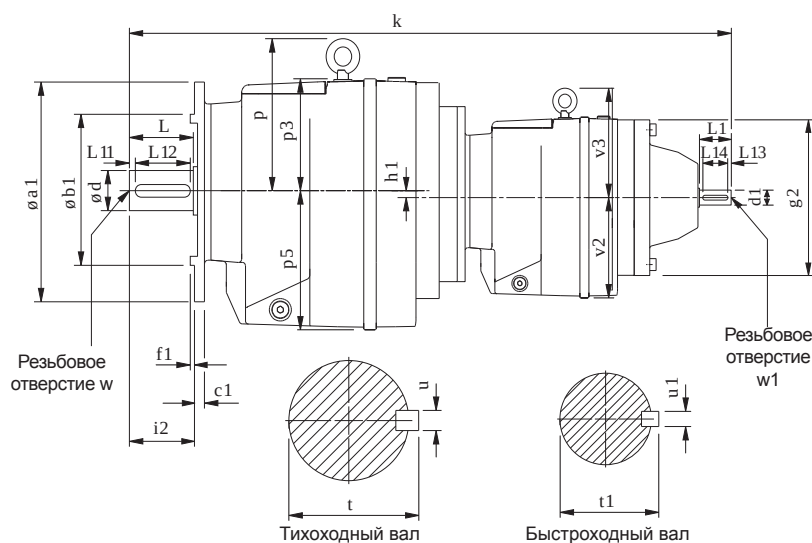
Типоразмеры 3, 4, 5, 6, 7 и 8
