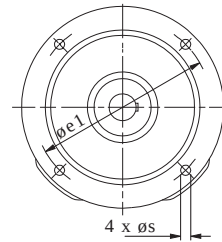
Типоразмеры 3, 4, 5, 7 и 8
