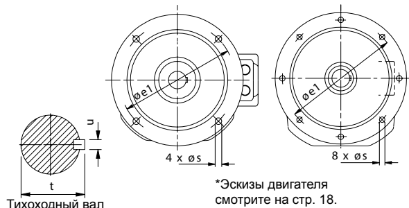
Типоразмеры 1, 2, 3, 4, 5, 6, 7 и 8
