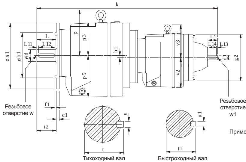
Типоразмеры 3, 4, 5, 7 и 8
