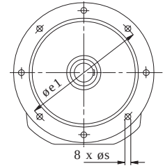
Типоразмеры 9, 10, 13 и 14
